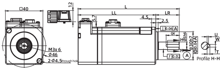
40mm flange
